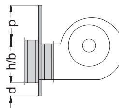
Торцевая стенка D с напорной стороны (h x b) положение вентилятора la
